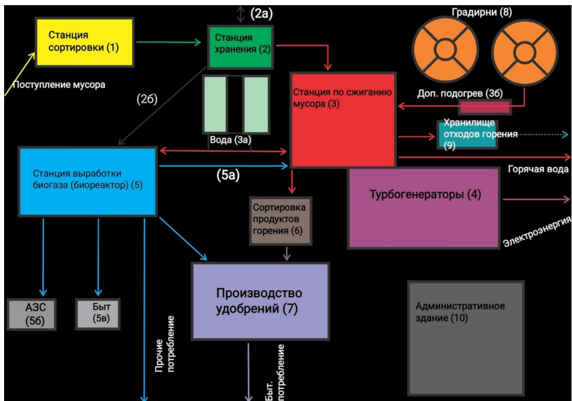
Рисунок 1 – План-схема станции по переработке органического мусора для использования продуктов переработки для получения электроэнергии
