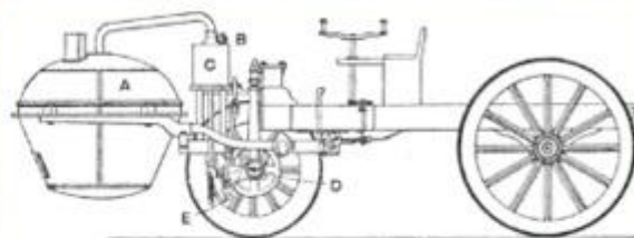
Чертёж Паровой телеги Кюньо (1769)
